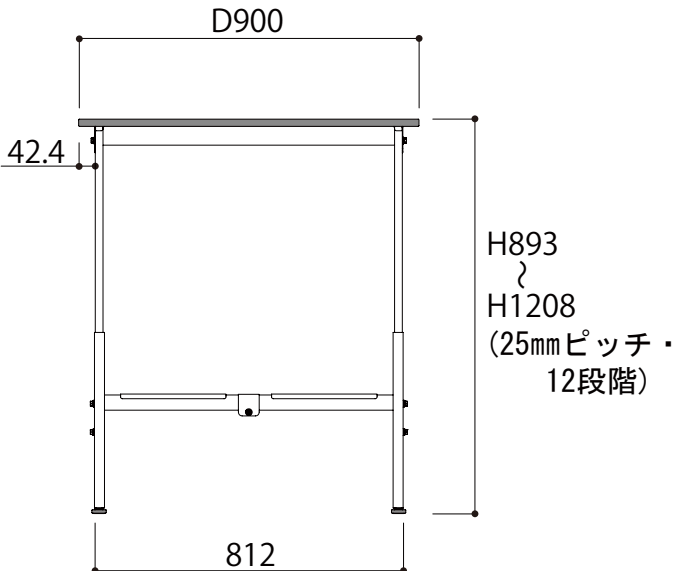
側面図
