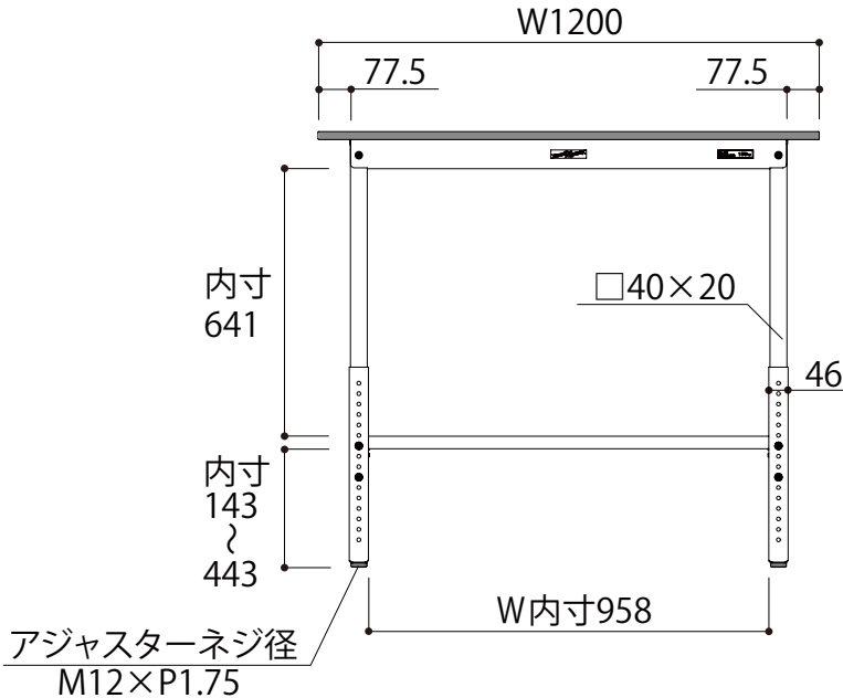
正面図
