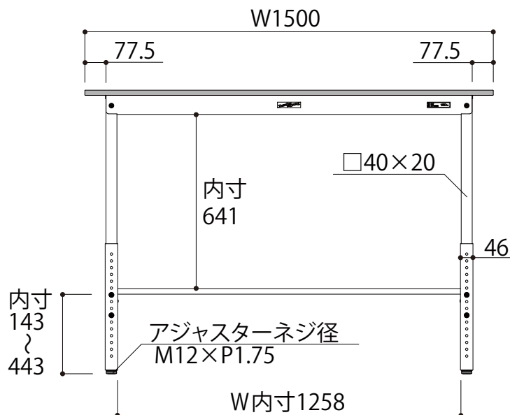
正面図
