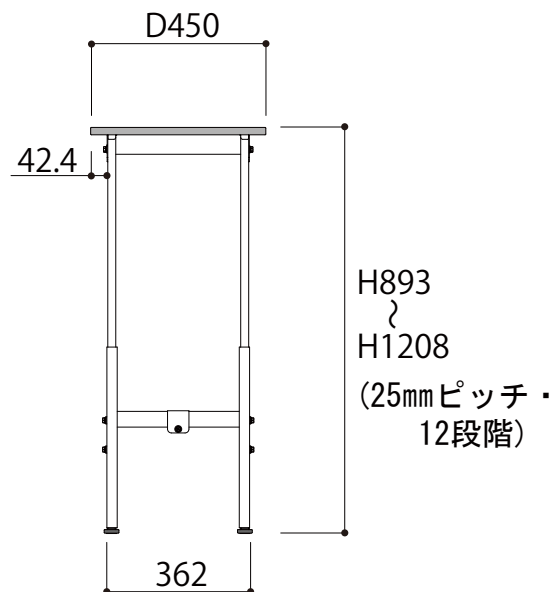
側面図
