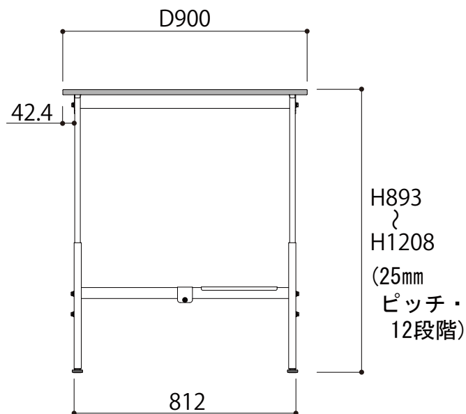
側面図
