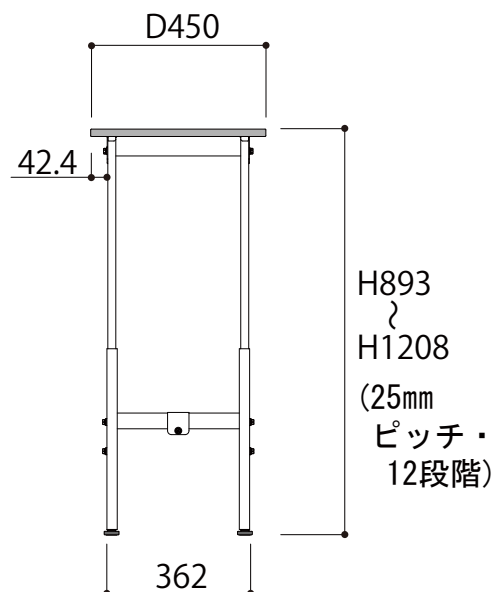
側面図
