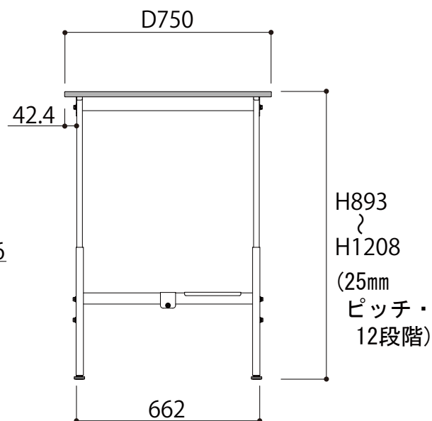
側面図
