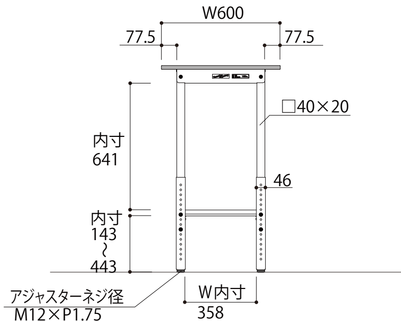
正面図
