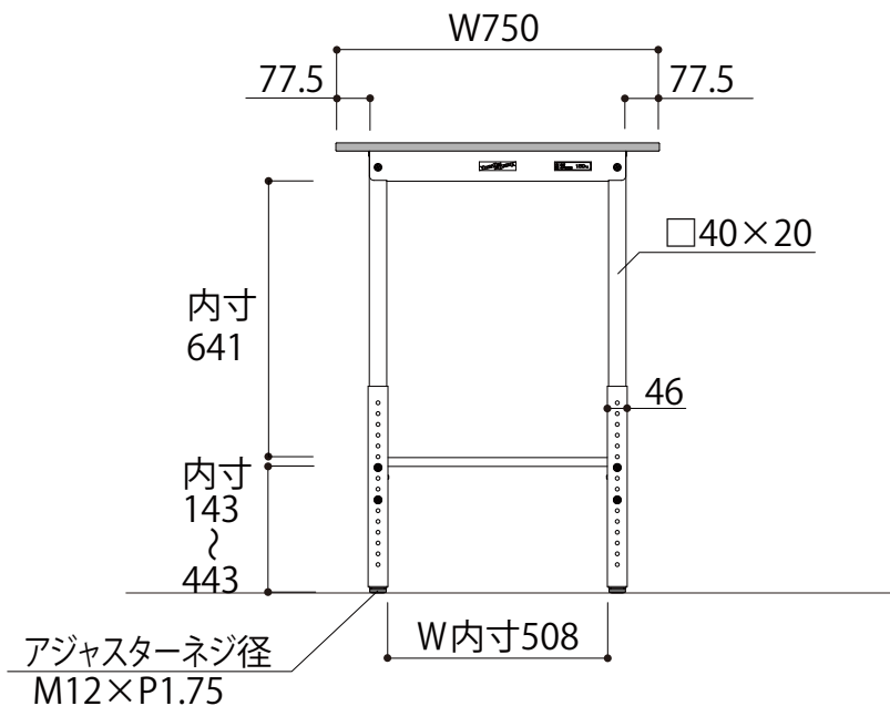
正面図
