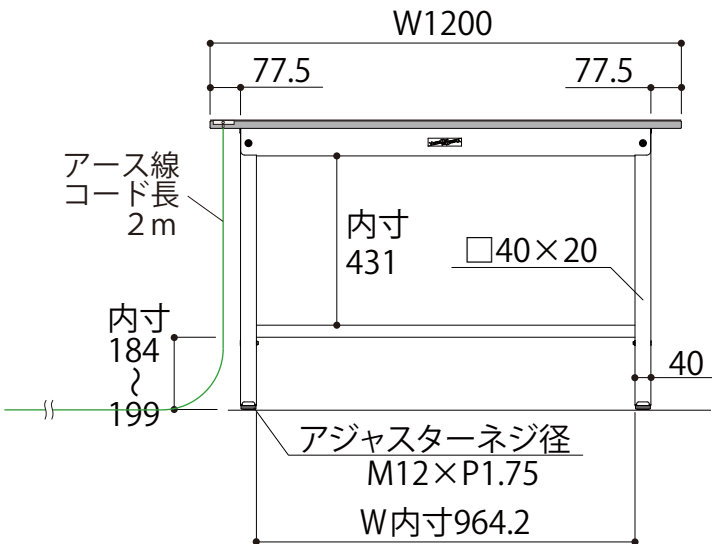
正面図
