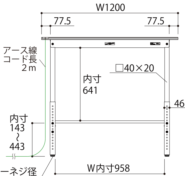
正面図
