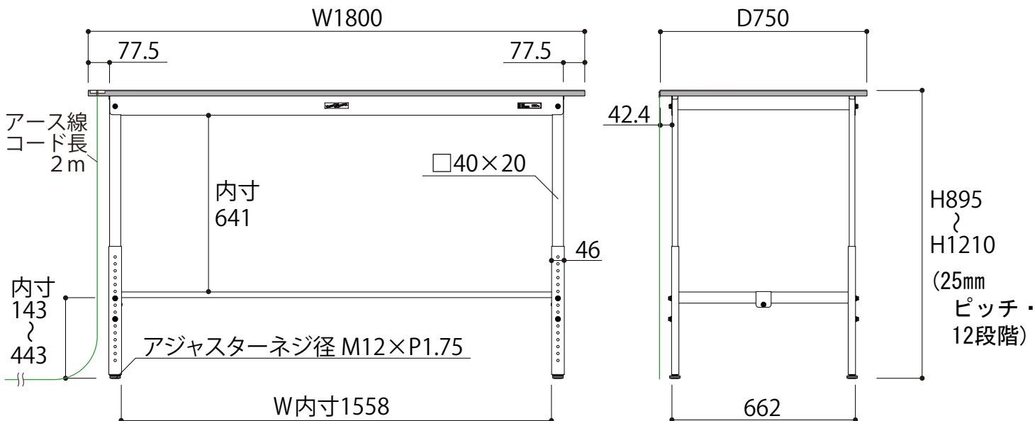
正面図
