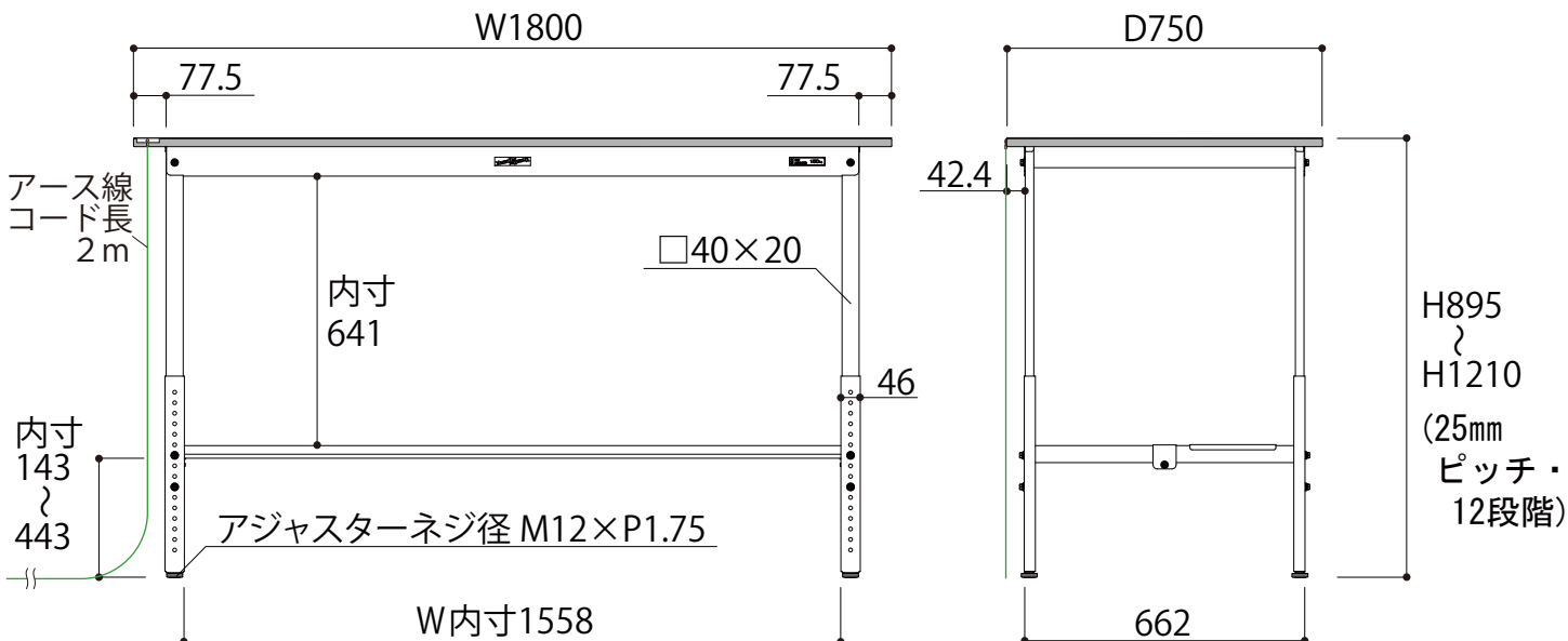
正面図
