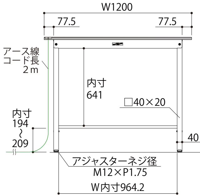
正面図
