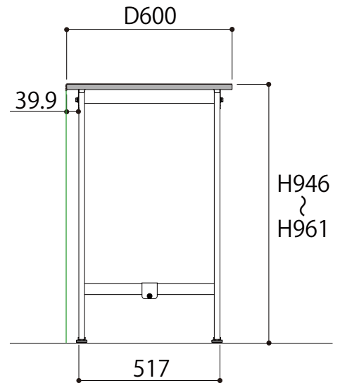
側面図
