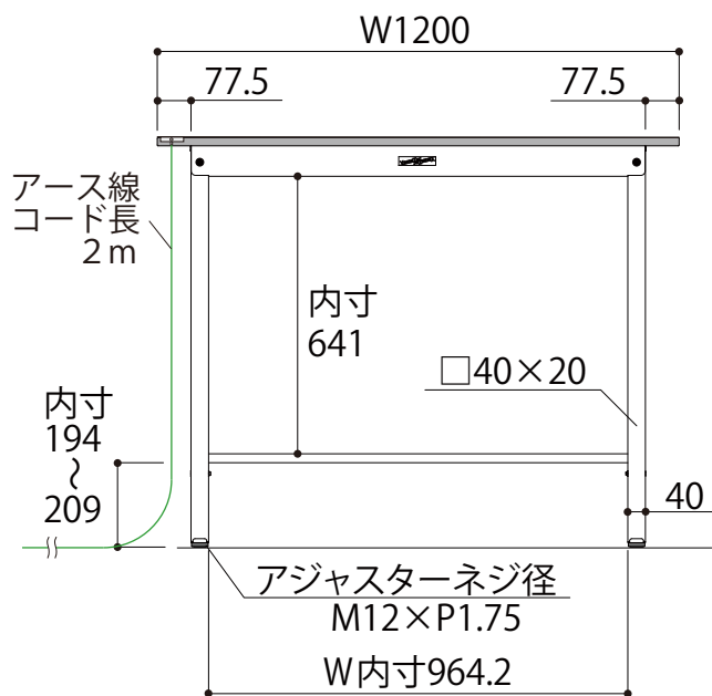
正面図
