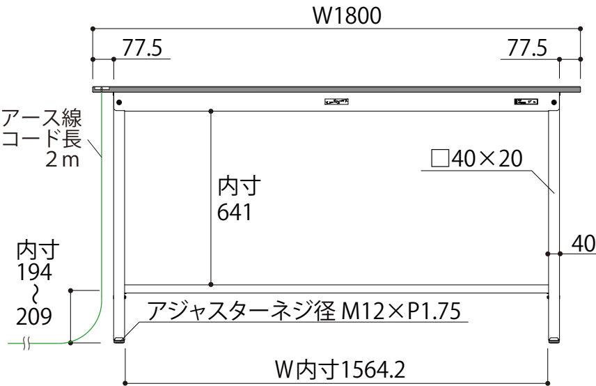
正面図
