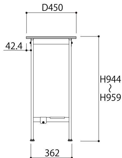
側面図
