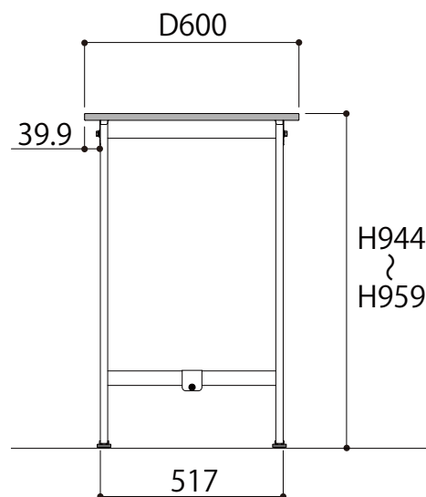
側面図
