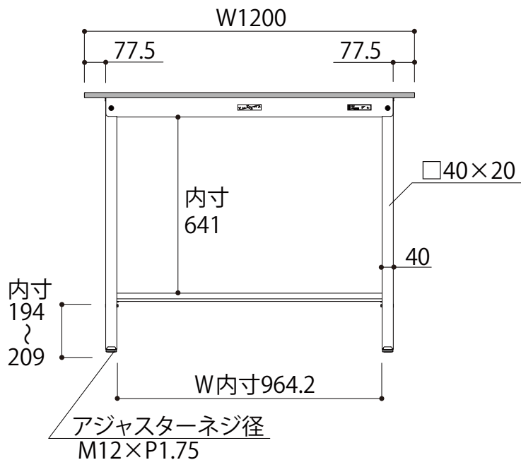
正面図
