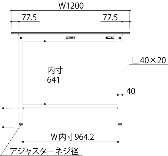
正面図
