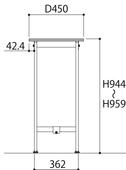
側面図
