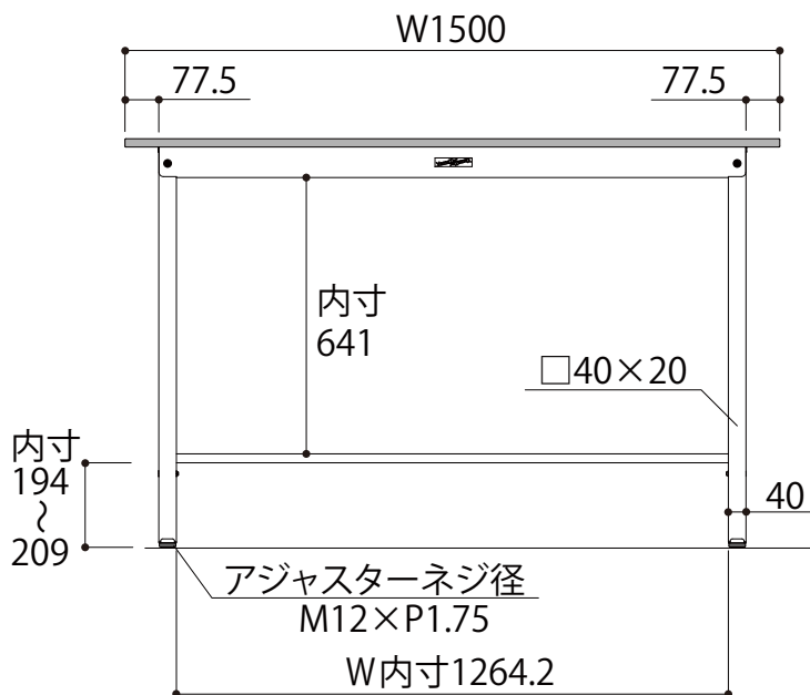
正面図
