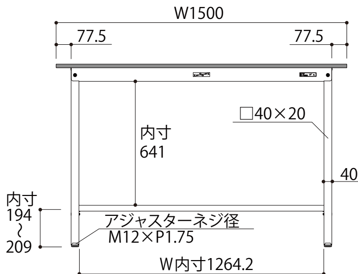
正面図
