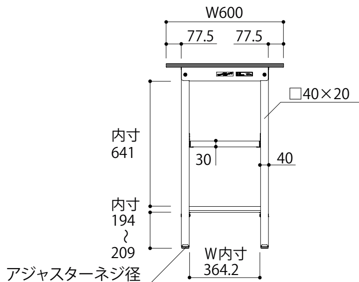
正面図
