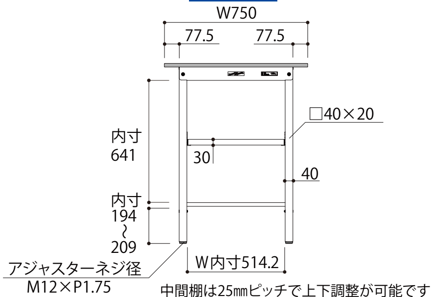
正面図
