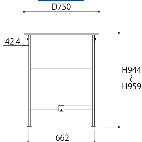
側面図
