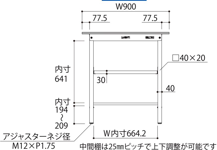
正面図
