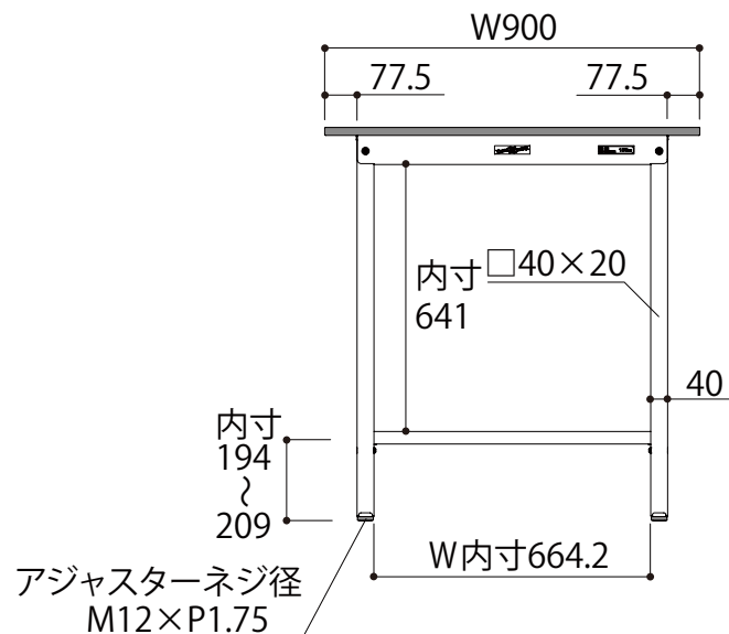
正面図
