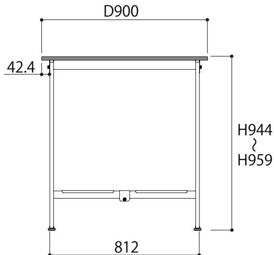
側面図
