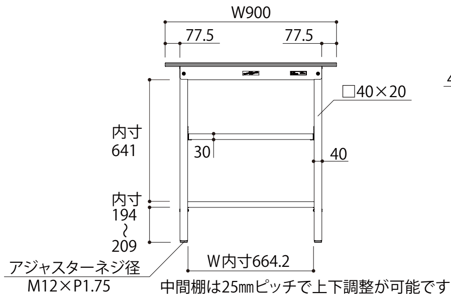
正面図
