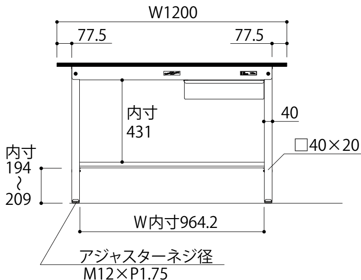
正面図
