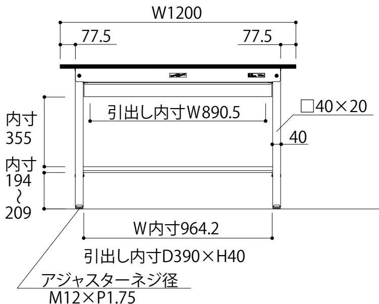
正面図
