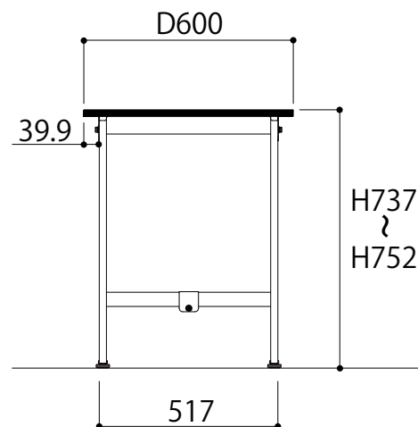
側面図
