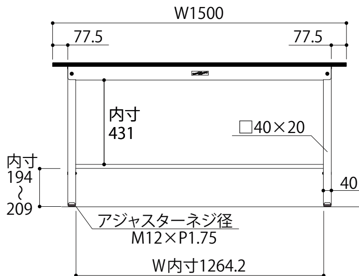
正面図
