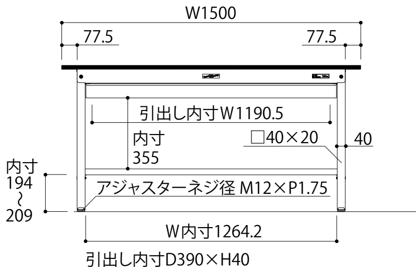
正面図
