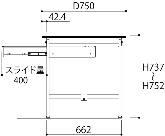
側面図
