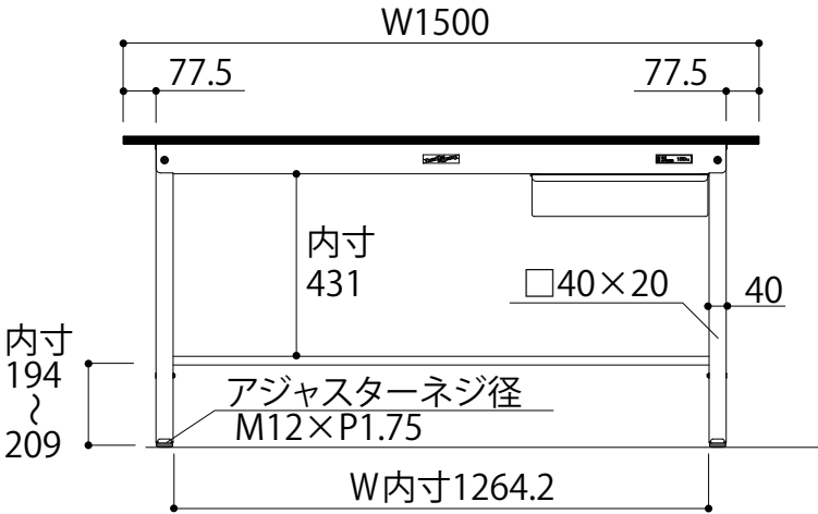
正面図
