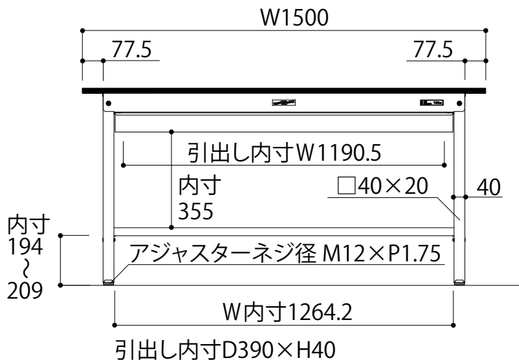
正面図
