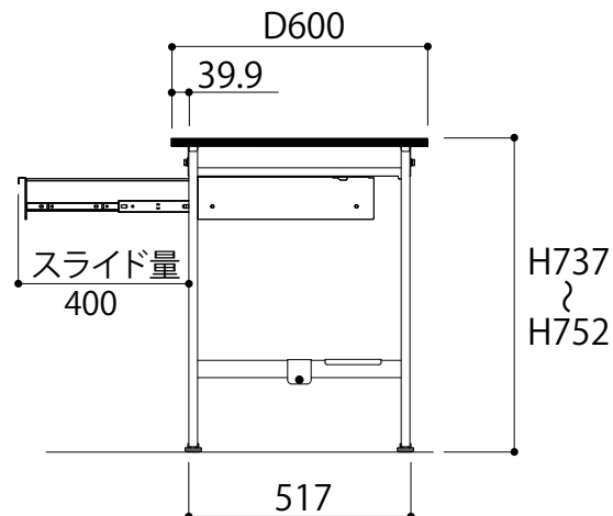
側面図
