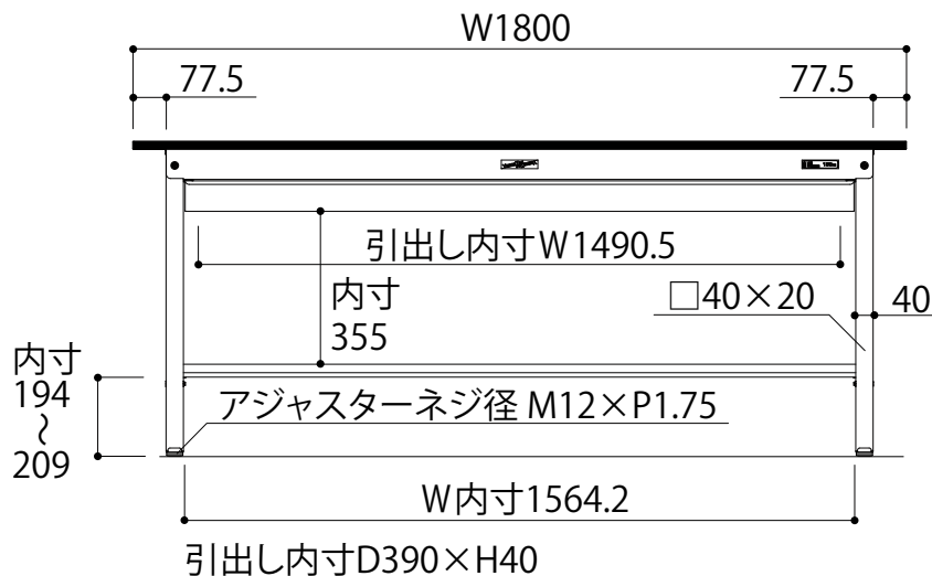
正面図
