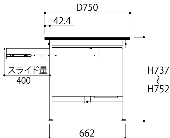
側面図
