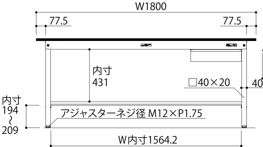
正面図
