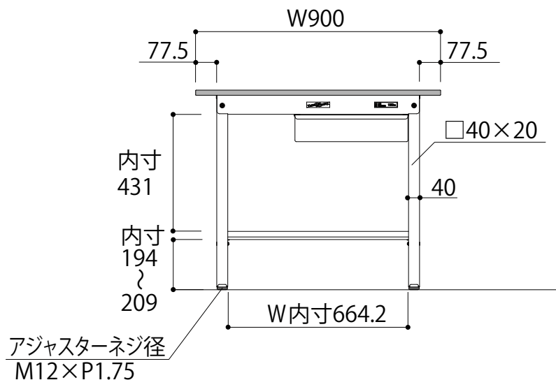
正面図
