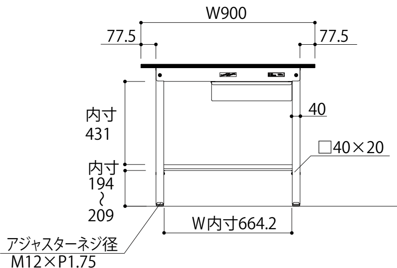
正面図
