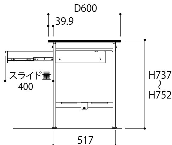
側面図
