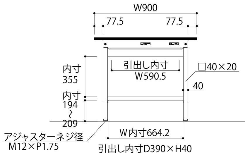
正面図
