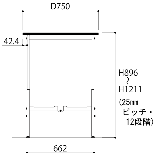
側面図
