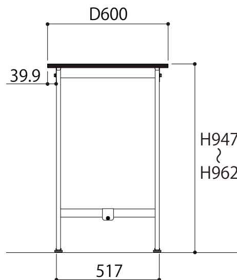
側面図
