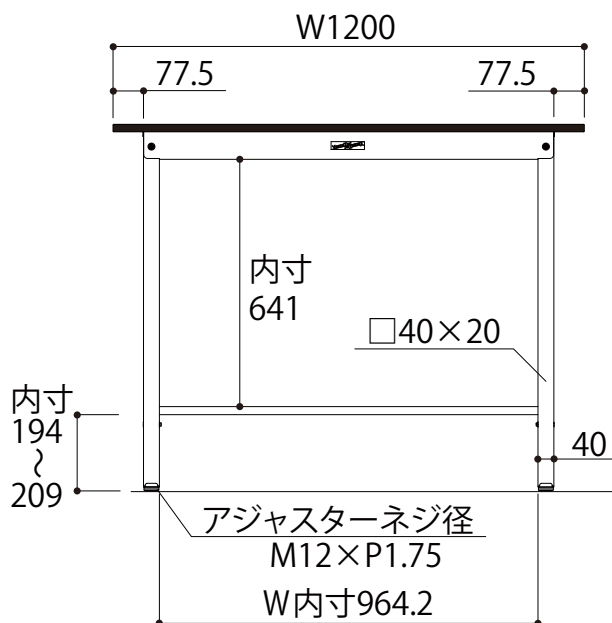
正面図
