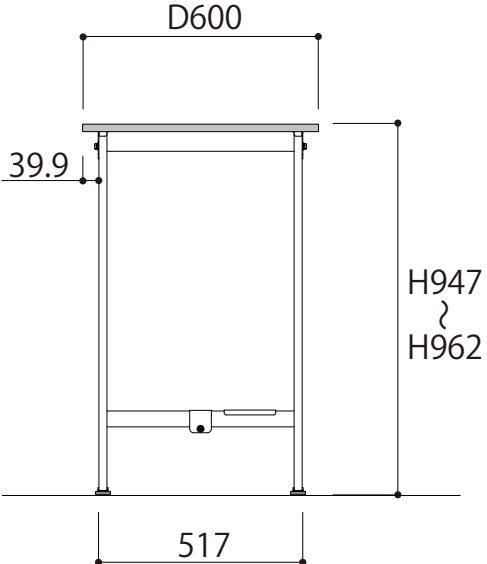
側面図
