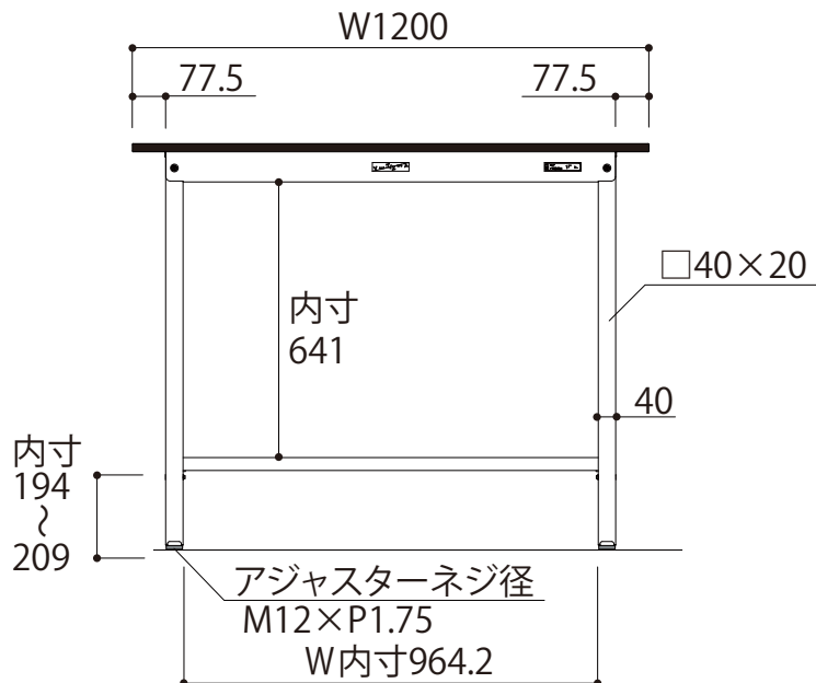
正面図
