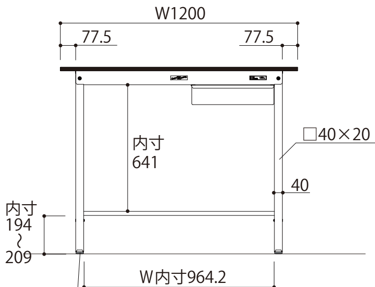
正面図
