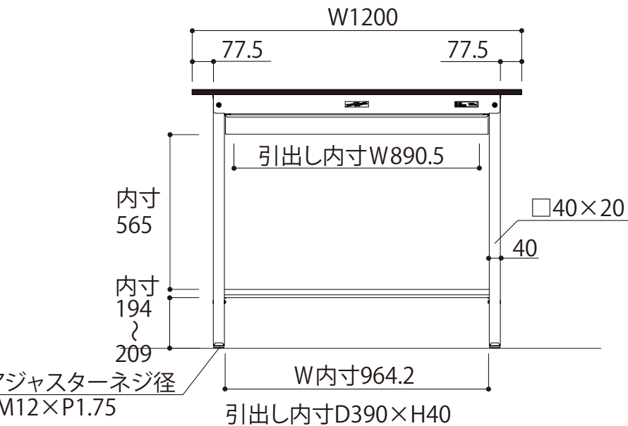
正面図
