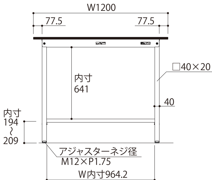
正面図
