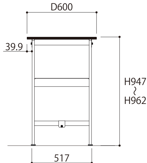
側面図
