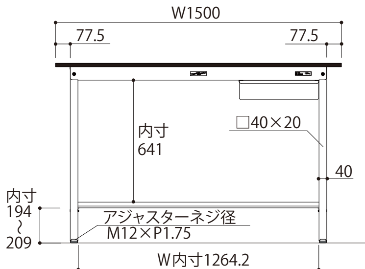
正面図
