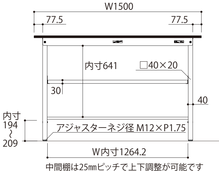
正面図
