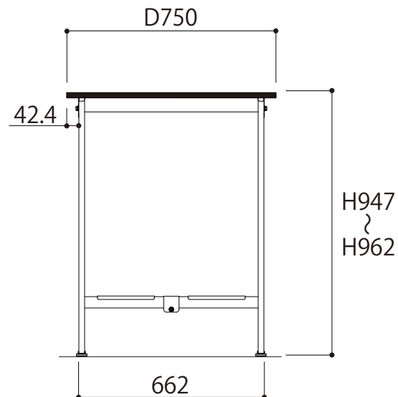
側面図
