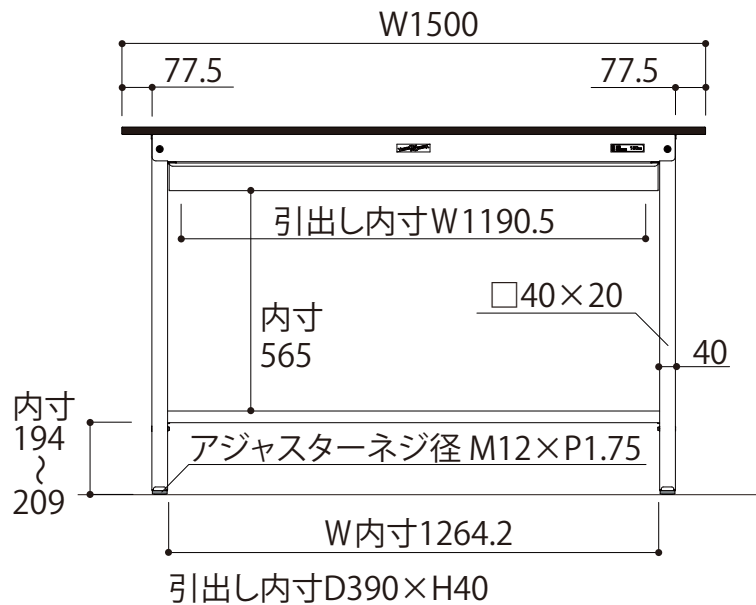
正面図
